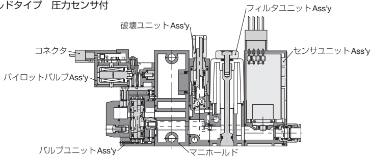
マニホールドタイプ 圧力センサ付
