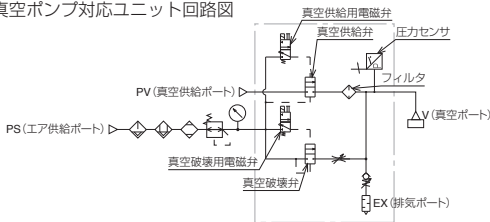
真空ポンプ対応ユニット回路図
