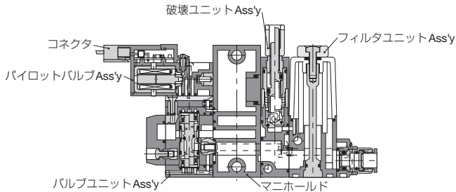
マニホールドタイプ 圧力センサ無し
