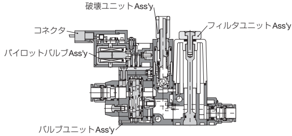
単体タイプ 圧力センサ無し
